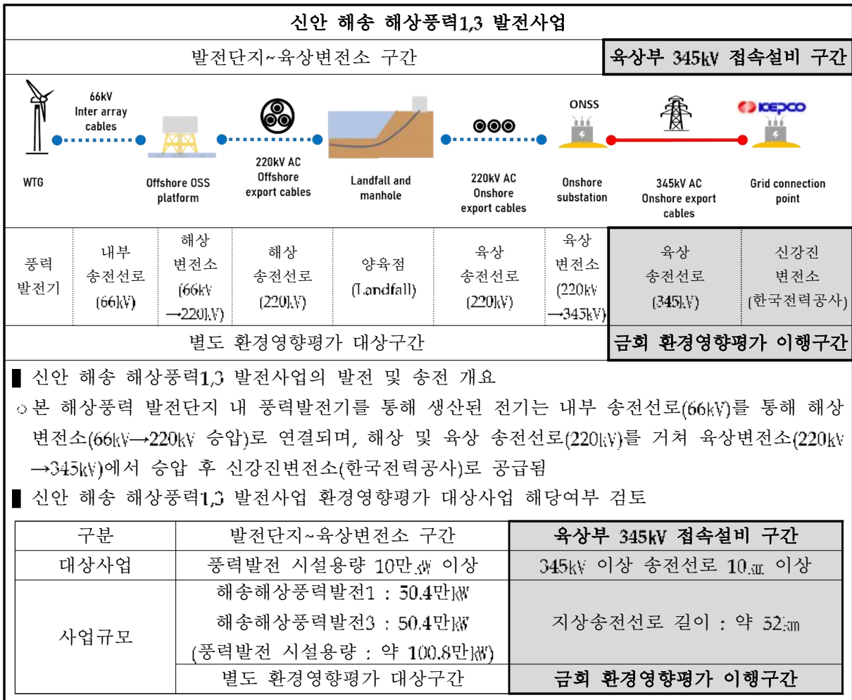
〈표 1.4-1〉 신안 해상 해상풍력1,3 발전사업 전체 구성도
